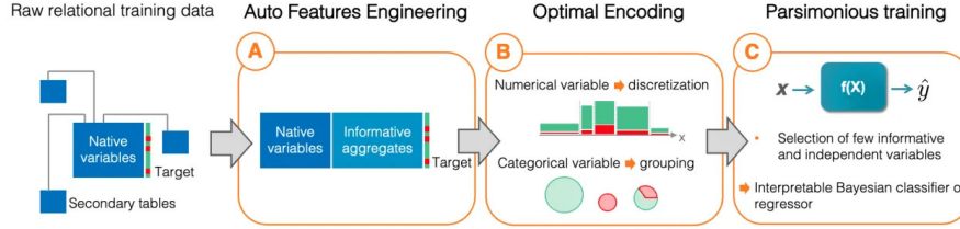
FIG. 1 – Processus d'apprentissage automatique implémenté par Khiops
