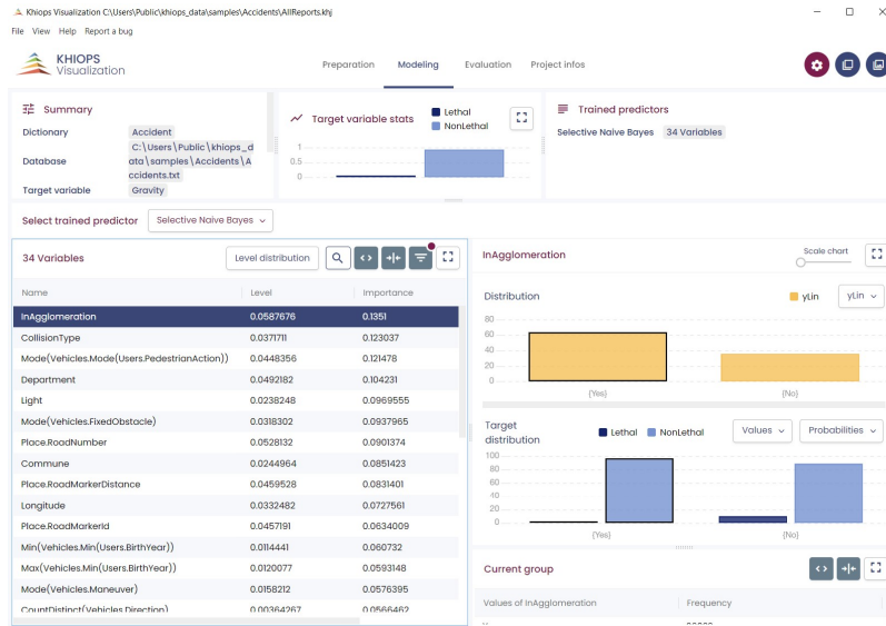
FIG. 4 – Capture d’écran de Khiops Visualisation après l’analyse de la base accidents et la construction de 100 agrégats
